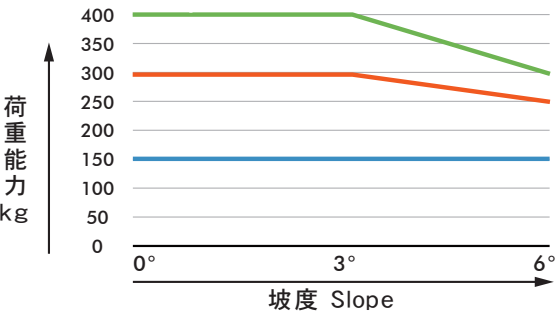
圖表： 坡度荷重能力 — MartinDrive (平台型) — MandyDrive (叉叉型) — WilsonXdrive (滾輪平台)
