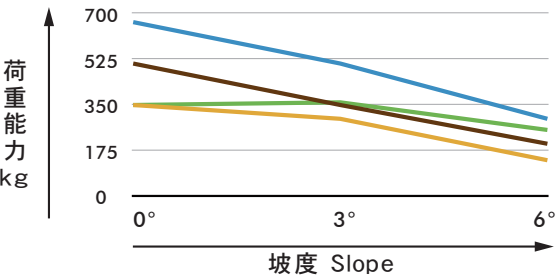
圖表： 坡度荷重能力 JustinGo (驅動輪OD200mm) JustinGo-AT (驅動輪OD250mm) JustinGoLift (驅動輪OD200mm) JustinGoLift-AT (驅動輪OD250mm)
