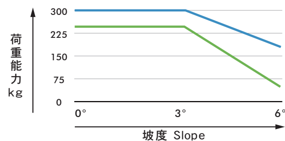
圖表： 坡度荷重能力 — MandyGo (牙叉型) — MandyGo-GT (卷料、桶料搬運車)
